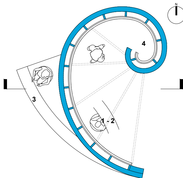
PIANTA
