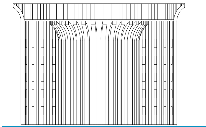
PROSPETTO SUD
