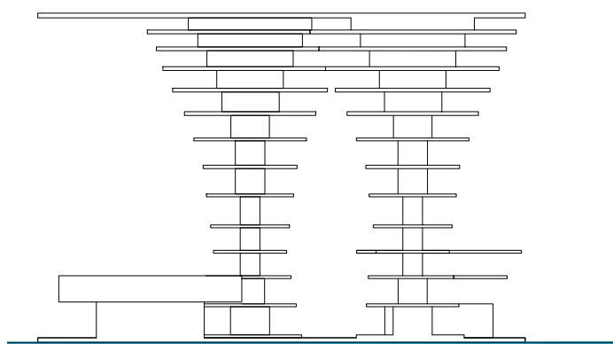
PROSPETTO SUD
