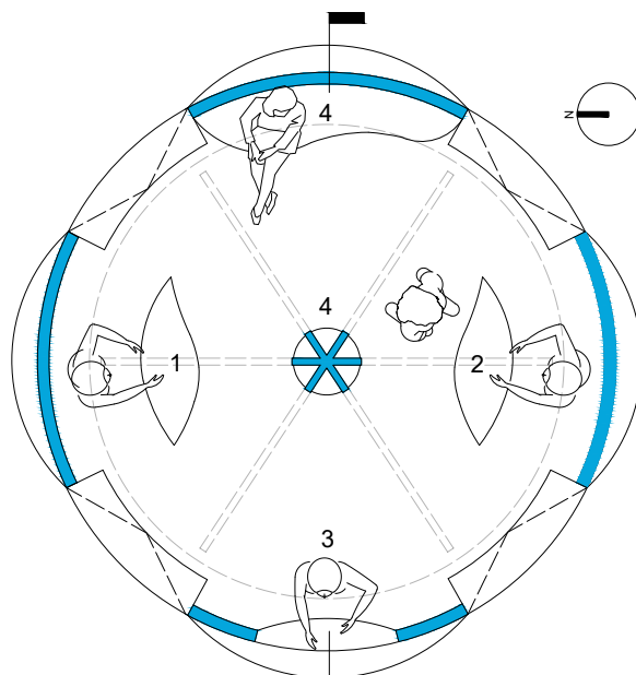
PIANTA
